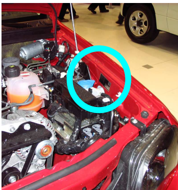
VIN PLATE LOCATION JIMNY
